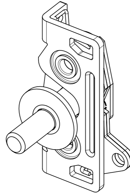
BOTTOM ACTUATION
