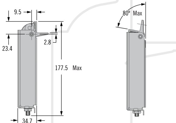
Posizione aperta
