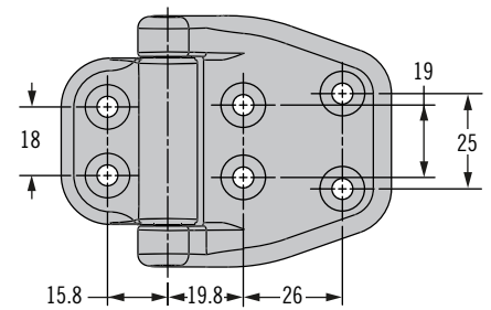
埋头通孔
